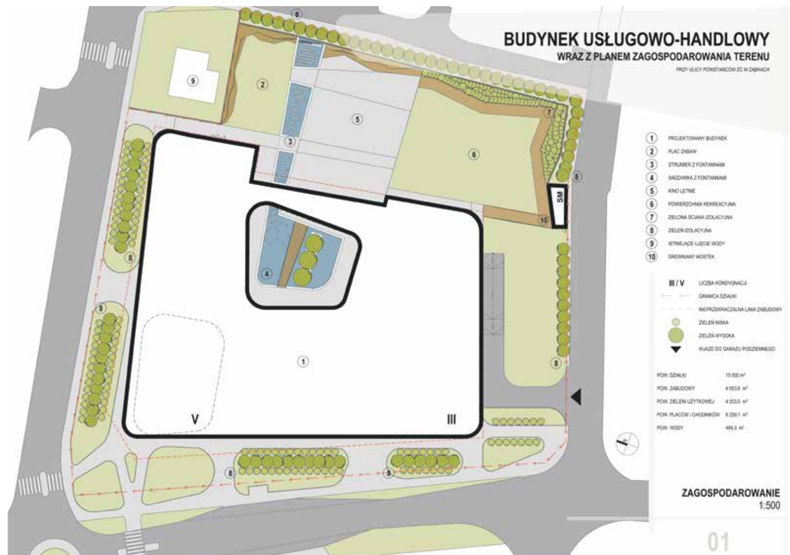
Koncepcja zagospodarowania całej działki po Gazomontażu
